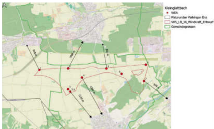
Layoutplanung für LB-16
